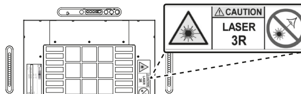
B Plassering av dekal klasse 3R laser, frittstående produkt
