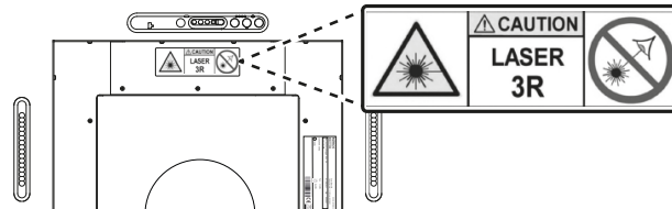
C Placering af mærkatklasse 3R laser, vægmonteret produkt
