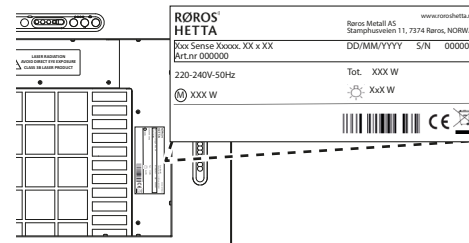
T Placering af typeskilt, vægmonteret produkt
