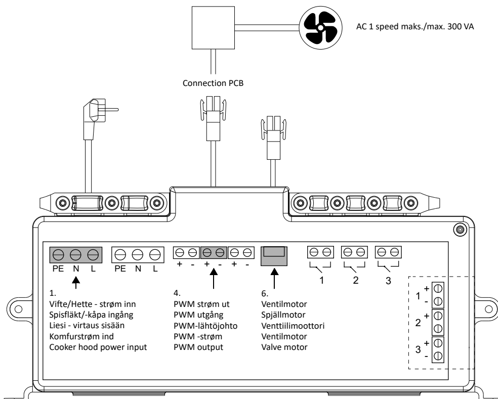
Koblingsskjema · Kopplingsdiagram · Yhteyskaavio · Tilslutningsordning · Connection Diagram
