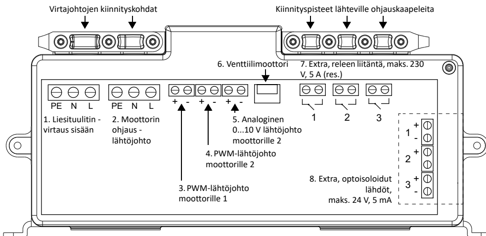
KytKentäkaavio PIO, vakio
